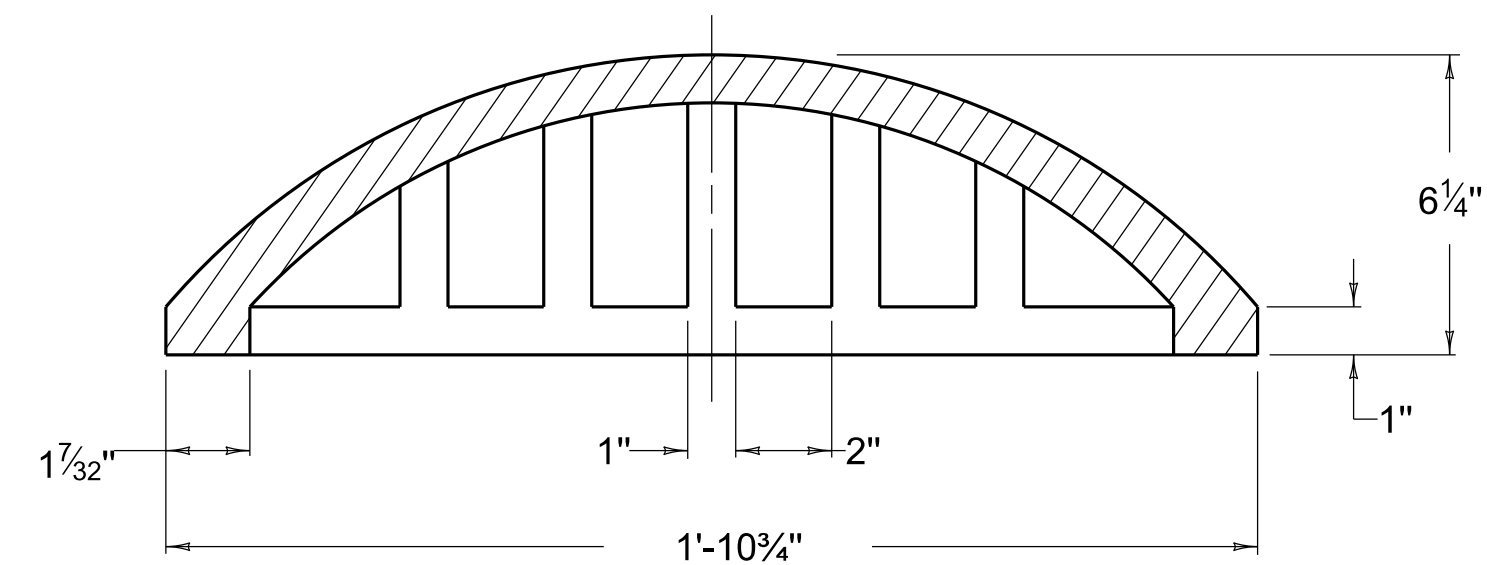
SECTION C-C TYPE 15 (BEEHIVE)
